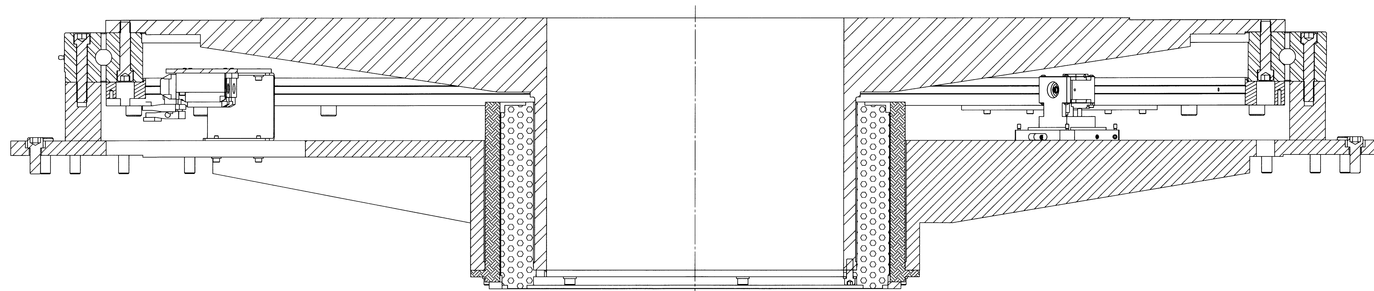
SECTION A-A SCALE 1 : 3
