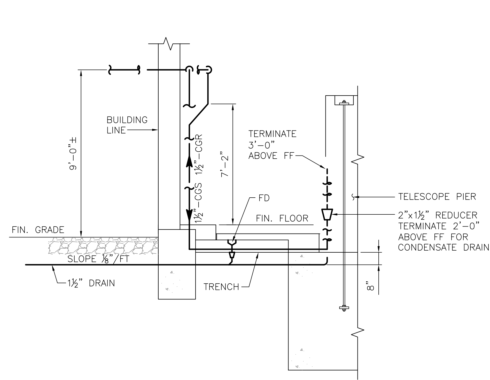
SECTION A SCALE: NTS
